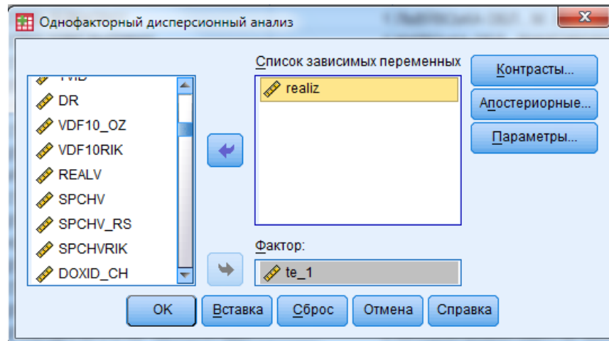
Рис. 2. Діалогове вікно "Однофакторний дисперсійний аналіз"
