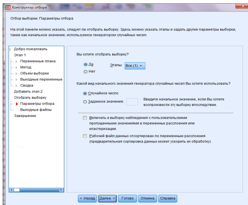
Рис. 23. Вибір параметрів відбору в діалоговому вікні "Конструктор відбору"
