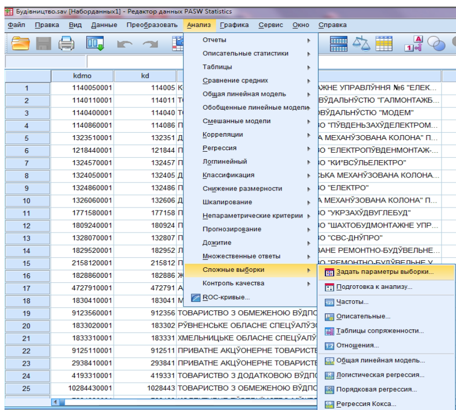
Рис. 16. Вибір у меню SPSS процедури "Складні вибірки"
